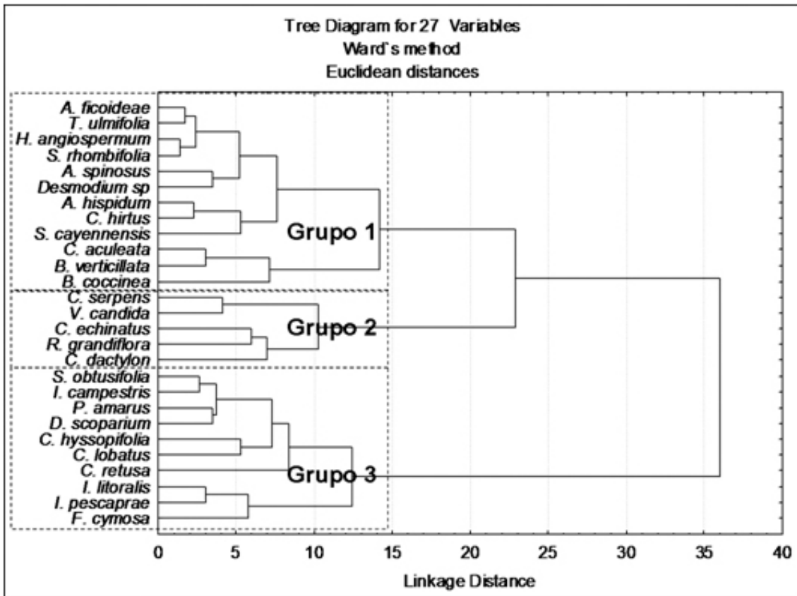
Figura 1. Grupos funcionais vegetais formados a partir de variações nos caracteres morfológicos foliares e fatores ecológicos das espécies encontradas na Praia de Boa Viagem, Recife, PE.
